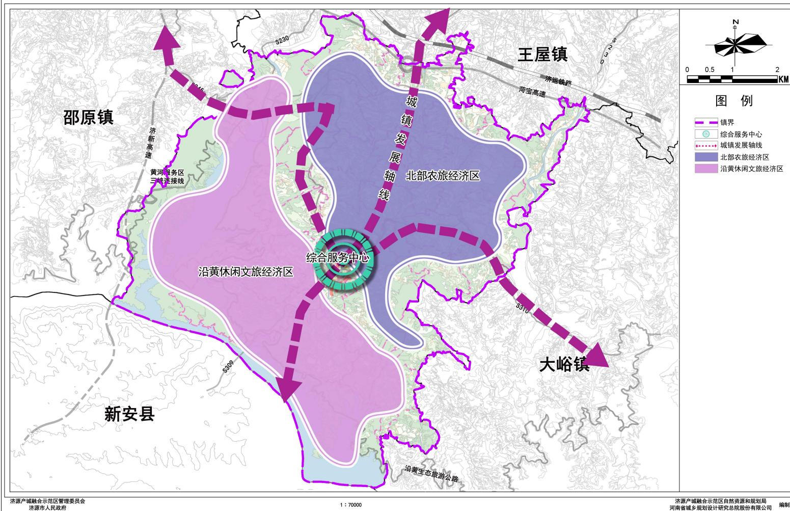
镇域国土空间总体格局规划图
